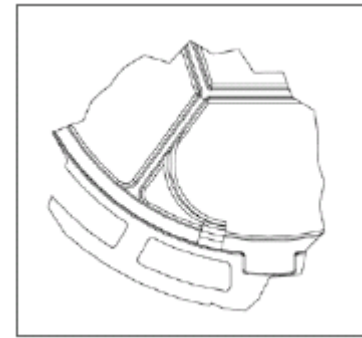
detail spodní strany víka
