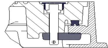
detail zámku
