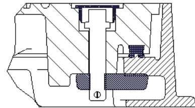
varianta – vestavění obrtlíkového zámku
