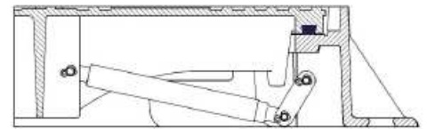
varianta – vestavění plynové vzpěry
